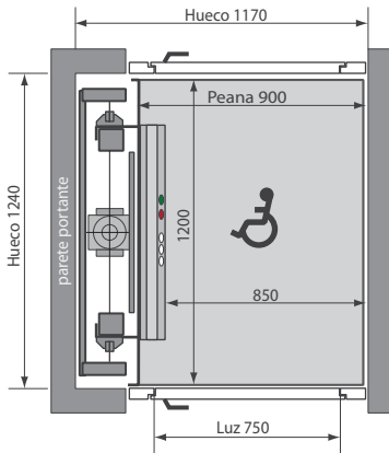
Plataforma con 2 accesos a 180°
