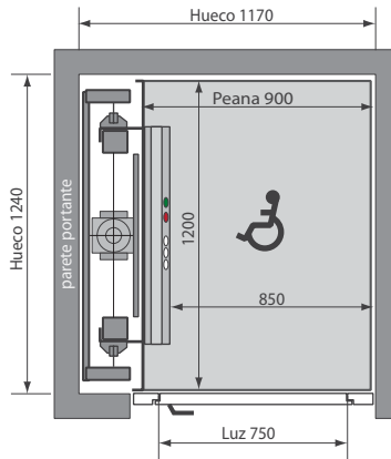
Plataforma con 1 acceso
