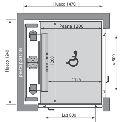
Plataforma con 2 accesos a 90°
